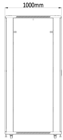
Vista lateral
